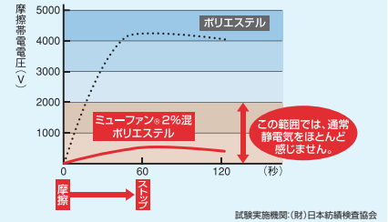
静電気除去性能 帯電防止機能テスト (測定条件20℃、40%RH)
